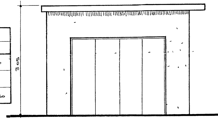
FACHADA GARAGE ESCALA 1.50
