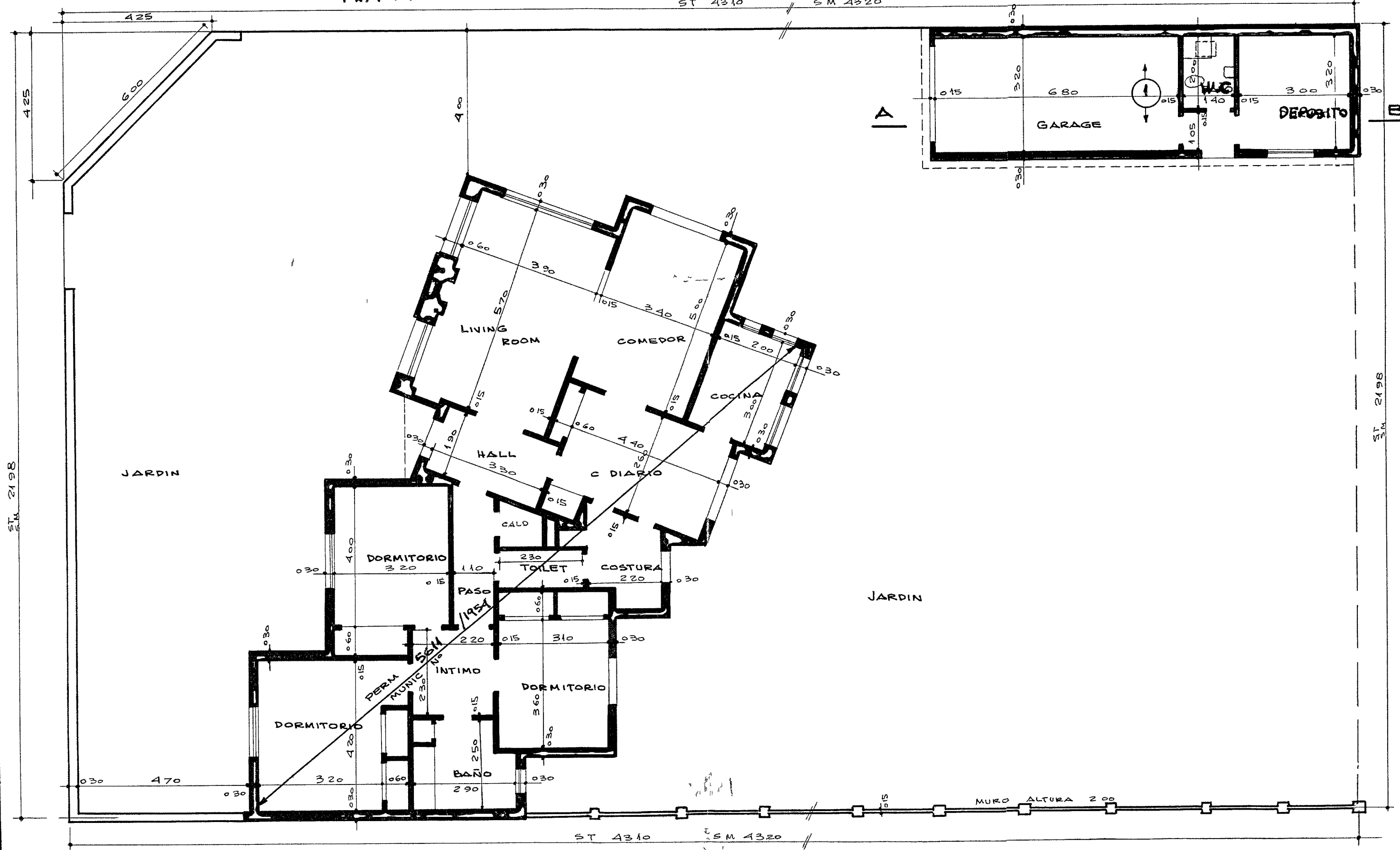
PLANTA ESCALA 1.00
